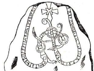
Snuggastenen R 8
